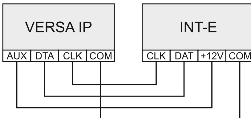
Рис. 11. Способ подключения модуля расширения INT-E к прибору.
