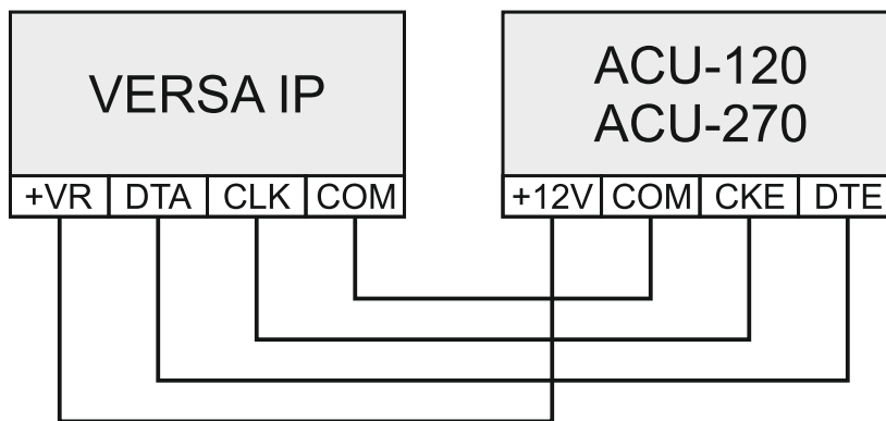
Рис. 7. Способ подключения контроллера ACU-120 / ACU-270 к прибору.
