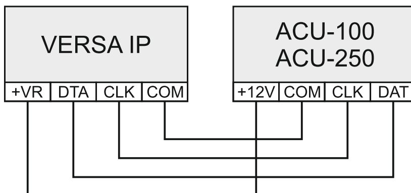
Рис. 8. Способ подключения контроллера ACU-100 / ACU-250 к прибору.
