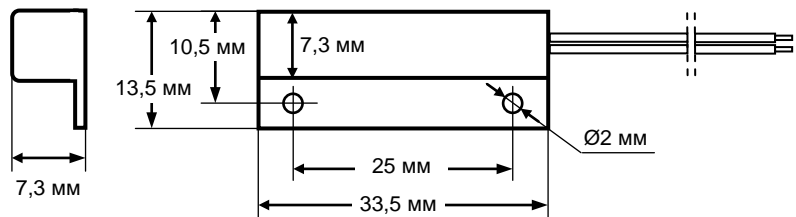
Рис. 1. Геркон извещателя К-1 2Е в пластмассовом корпусе
