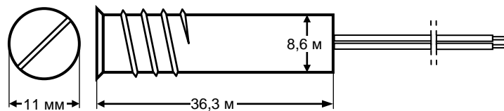
Рис. 3. Геркон извещателя К-3 2Е в металлическом корпусе
