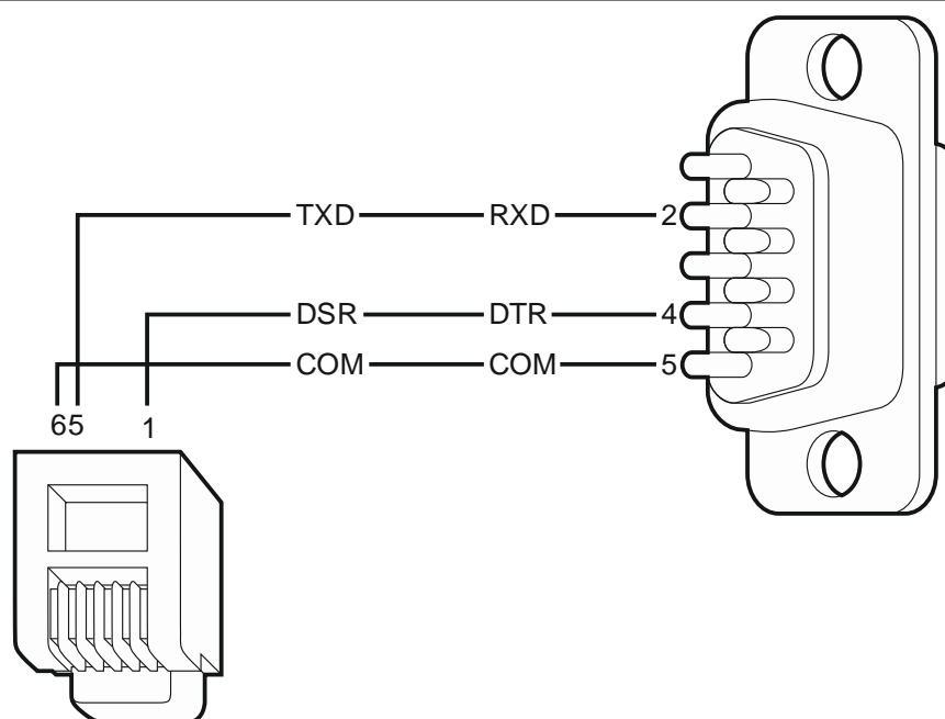
Рис. 19. Способ подключения принтера с помощью штекера DB-9 тип «папа» (вид со стороны точек пайки). С левой стороны – штекер RJ, подключаемый к разъему на плате прибора.
