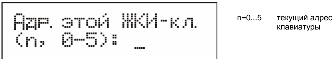
Рис. 23. Настройка адреса ЖКИ-клавиатуры.
