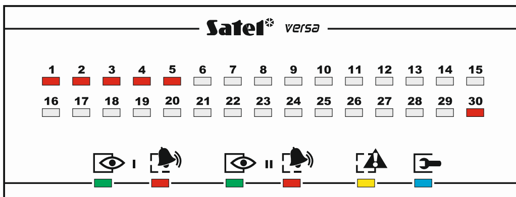
Рис. 24. Настройка адреса светодиодной клавиатуры. Для отображения адреса используются светодиоды с цифрами от 1 до 5 и 30 (адрес 0). Светодиод, отвечающий установленному адресу, быстро мигает, а остальные светодиоды горят.
