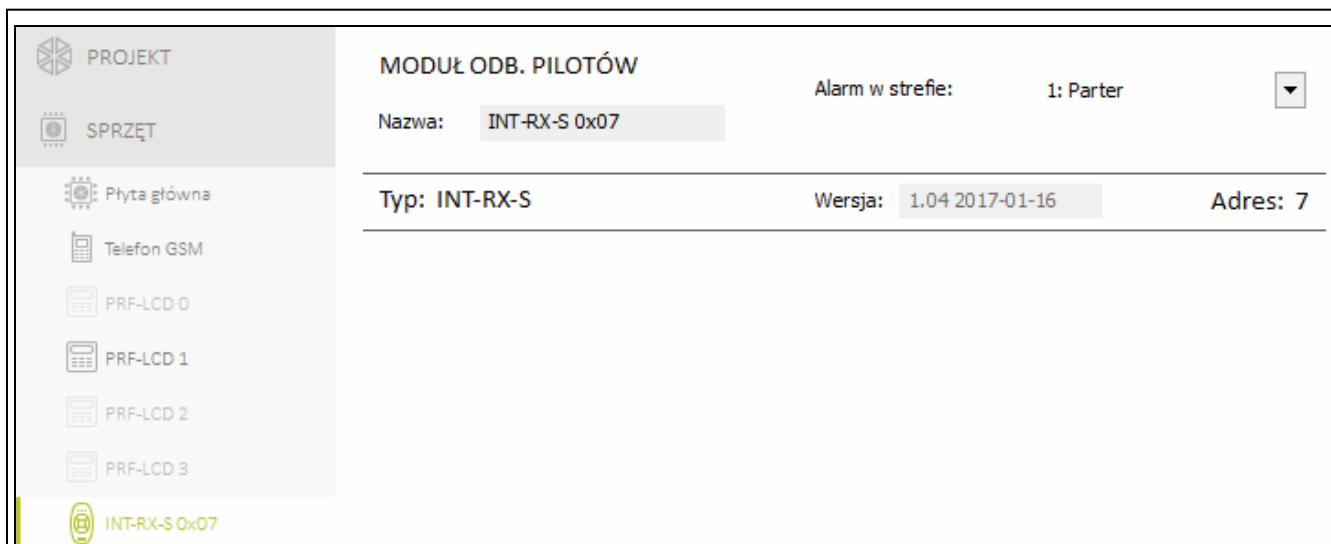
Rys. 9. Zakładka z ustawieniami ekspandera obsługi pilotów 433 MHz.
