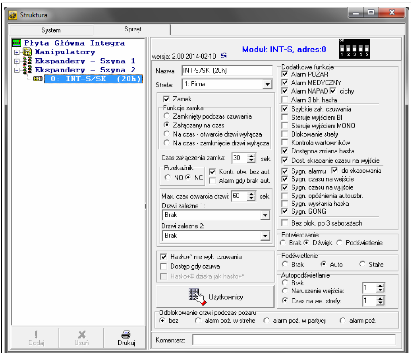
Rys. 5. Program DloadX: parametry i opcje klawiatury strefowej.
