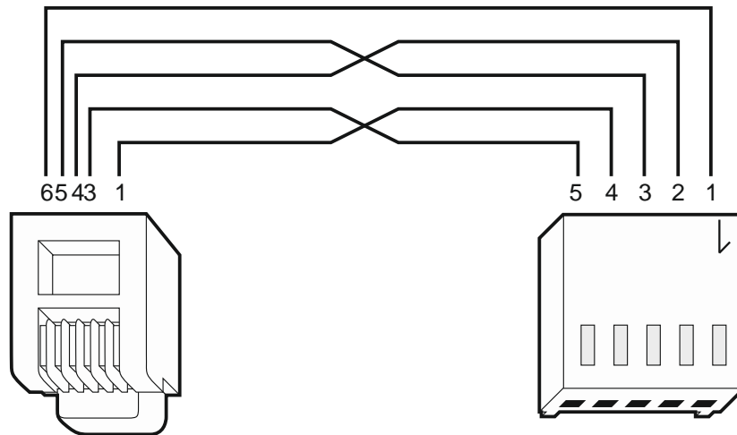
Fig. 17. Aansluiting van de RS-232 poorten van het alarmsysteem en extern modem met de PIN5 aansluiting (de door SATEL gemaakte ETHM-1 / ETHM-1 Plus en GSM modules worden op dezelfde manier aangesloten). Links weergegeven is de RJ connector welke aangesloten wordt op de RJ aansluiting van de hoofdprint. Rechts weergegeven is de PIN5 stekker. Een kant en klare kabel is bij Osec verkrijgbaar (RJ/PIN5).
