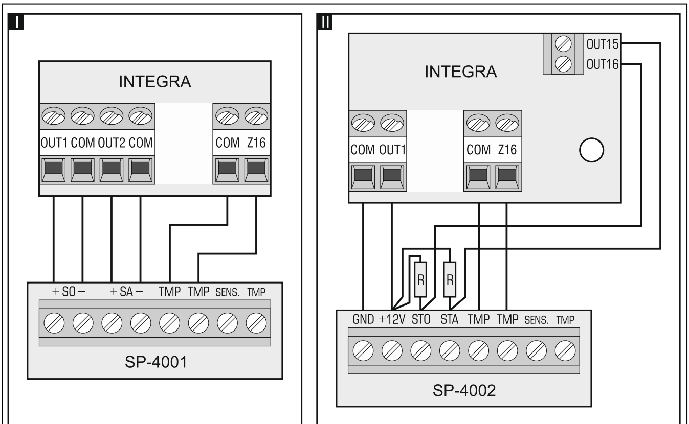
Fig. 11. Sirene aansluitvoorbeeld. I – sirene zonder eigen voeding – alarm signalering wordt aangestuurd door de hoogvermogen uitgangen. II - sirene met eigen voeding – alarm signalering wordt aangestuurd door de laagvermogen uitgangen waarbij de hoogvermogen uitgang dient als voedingsuitgang. De weerstandswaarde van R is 2.2 kΩ. In beide gevallen is de sabotage aangesloten op zone Z16.
