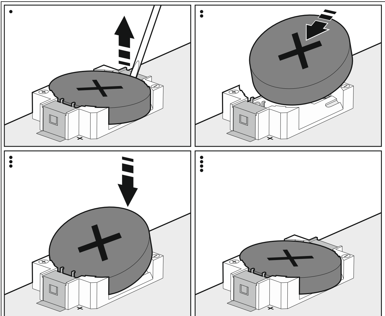
Fig. 19. Vervangen van de batterij op een INTEGRA 32 / INTEGRA 64 / INTEGRA 128 alarmsysteem.
