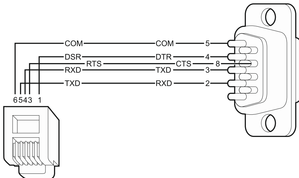
Fig. 11. Computer aansluiting via de RS-232 poort. Links weergegeven is de RJ connector welke aangesloten wordt op de RJ aansluiting van de hoofdprint. Rechts weergegeven is de DB-9 female connector (aanzicht soldeer zijde). Een kant en klare programmeerkabel is te verkrijgen onder de benaming DB9F/RJ-KPL set.
