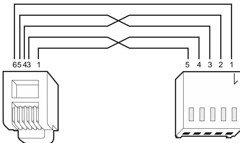
Fig. 13. Aansluiting van de RS-232 poorten van het alarmsysteem en het modem met een PIN5 aansluiting (de door SATEL gemaakte ETHM-1 / ETHM-1 Plus en GSM modules worden op dezelfde manier aangesloten). Links weergegeven is de RJ connector welke aangesloten wordt op de RJ aansluiting van de hoofdprint. Rechts weergegeven is de PIN5 stekker. Een kant en klare kabel is verkrijgbaar bij Osec (RJ/PIN5).
