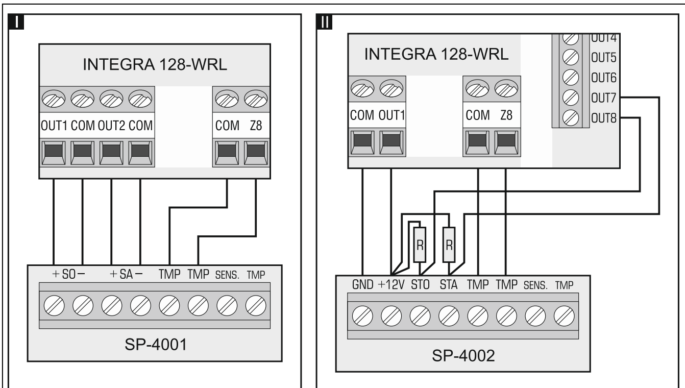
Fig. 9. Sirene aansluit voorbeeld. I – sirene zonder eigen voeding – alarm signalering wordt aangestuurd door de hoogvermogen uitgangen. II - sirene met eigen voeding – alarm signalering wordt aangestuurd door de laagvermogen uitgangen waarbij de hoogvermogen uitgang dient als voedingsuitgang. De weerstandswaarde van R is 2.2 k \Omega . In beide gevallen is de sabotage aangesloten op zone Z8.
