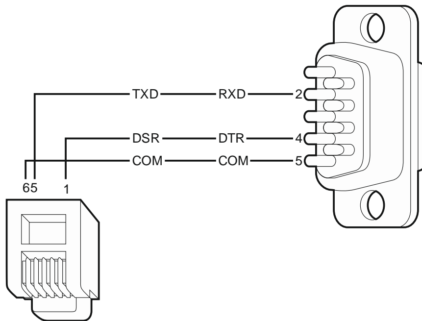
Fig. 15. Printer aansluiting met gebruik van de DB-9 male plug (aanzicht soldeerzijde). Links weergegeven is de RJ connector welke aangesloten wordt op de RJ aansluiting van de hoofdprint.
