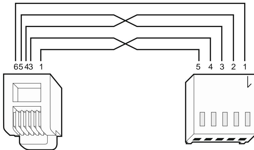
Fig. 15. Aansluiting van de RS-232 poorten van het alarmsysteem en het modem met een PIN5 aansluiting (de door SATEL gemaakte ETHM-1 / ETHM-1 Plus en GSM modules worden op dezelfde manier aangesloten). Links weergegeven is de RJ connector welke aangesloten wordt op de RJ aansluiting van de hoofdprint. Rechts weergegeven is de PIN5 stekker. Een kant en klare kabel is verkrijgbaar bij Osec (RJ/PIN5).
