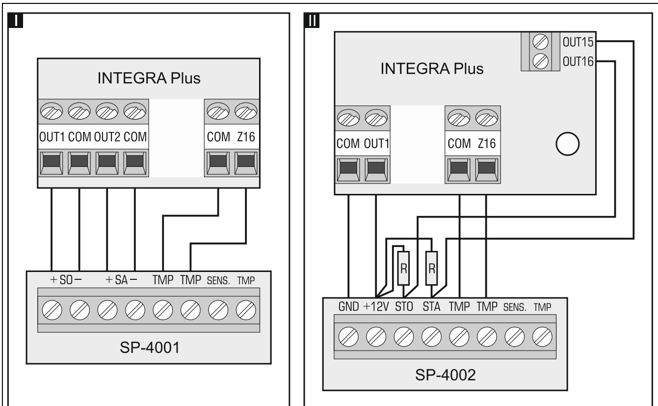
Fig. 9. Sirene aansluit voorbeeld. I – sirene zonder eigen voeding – alarm signalering wordt aangestuurd door de hoogvermogen uitgangen. II - sirene met eigen voeding – alarm signalering wordt aangestuurd door de laagvermogen uitgangen waarbij de hoogvermogen uitgang dient als voedingsuitgang. De weerstandswaarde van R is 2.2 k \Omega . In beide gevallen is de sabotage aangesloten op zone Z16.
