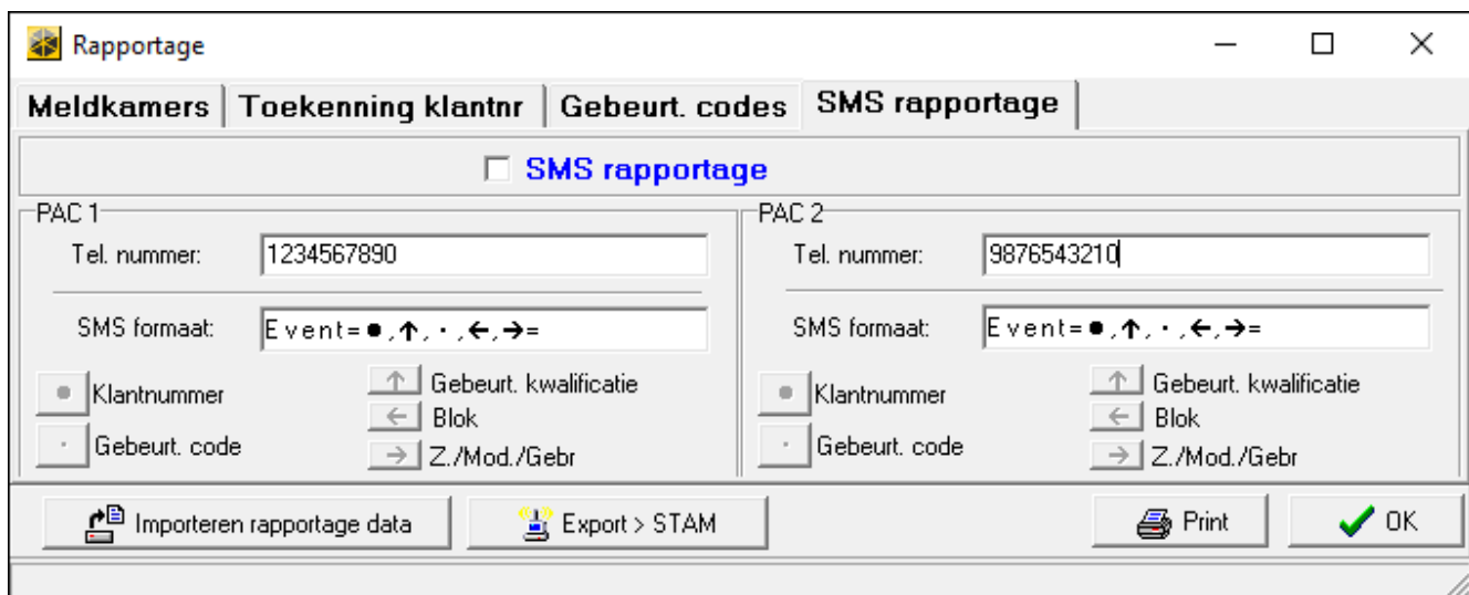
Fig. 12. Voorbeeld van meldkamer instellingen in het DLOADX programma.
