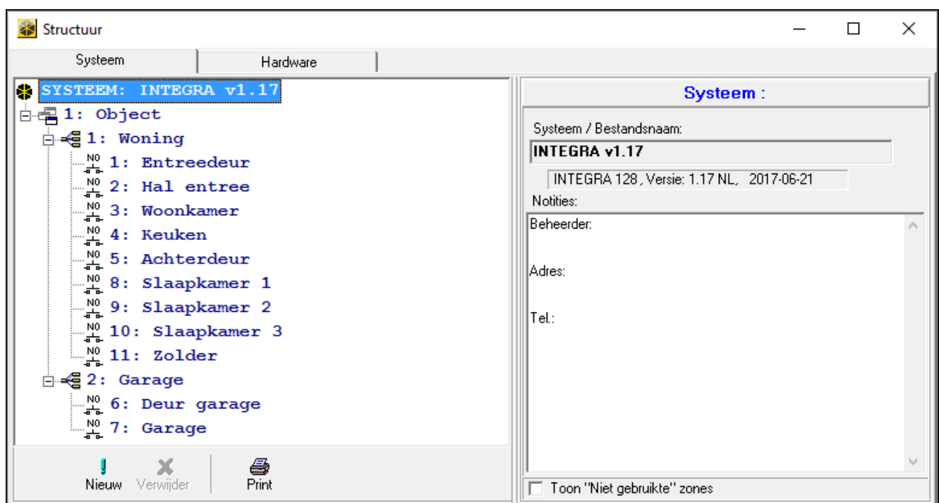
Fig. 2. Voorbeeld van de systeemstructuur in het DLOADX programma.
