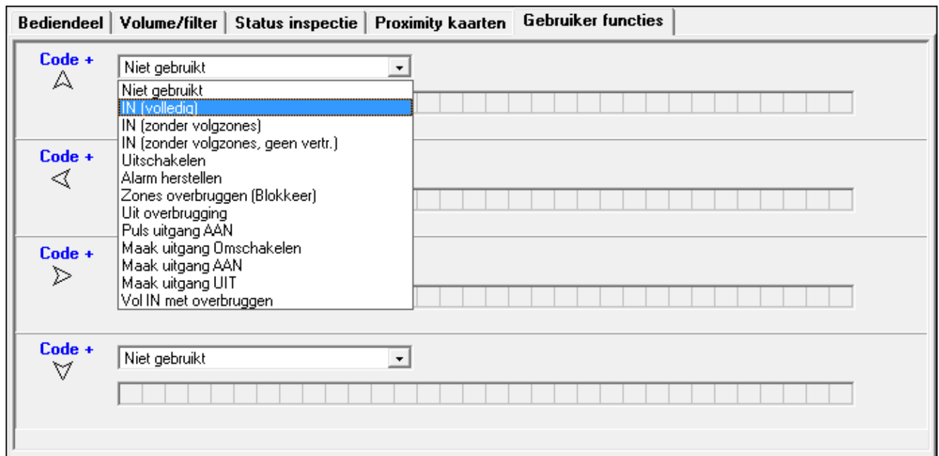
Fig. 10. “Gebruiker functies” tabblad in het DLOADX programma.
