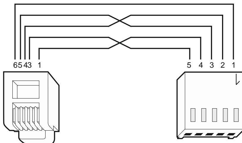
Fig. 13. Aansluiting van de RS-232 poorten van het alarmsysteem en het modem met een PIN5 aansluiting (de door SATEL gemaakte ETHM-1 / ETHM-1 Plus en GSM modules worden op dezelfde manier aangesloten). Links weergegeven is de RJ connector welke aangesloten wordt op de RJ aansluiting van de hoofdprint. Rechts weergegeven is de PIN5 stekker. Een kant en klare kabel is verkrijgbaar bij Osec (RJ/PIN5).
