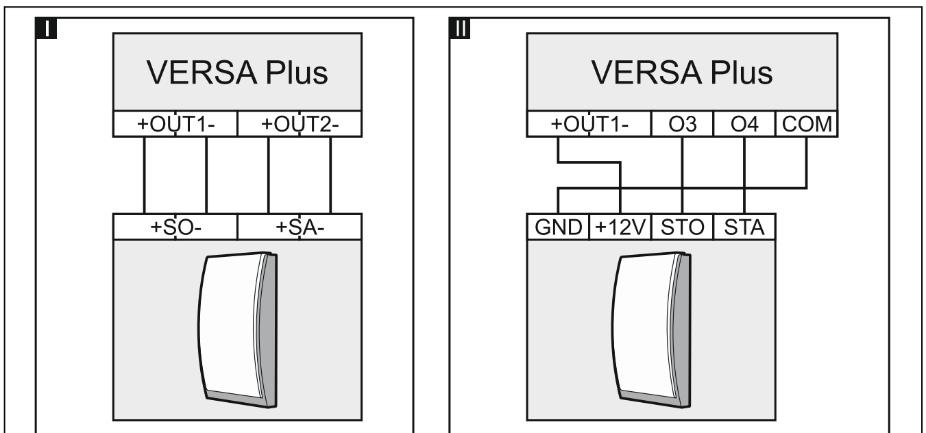
Fig. 18. Mode de raccordement de la sirène aux sorties de la centrale. I – sirène sans sa propre alimentation. II – sirène avec sa propre alimentation.
