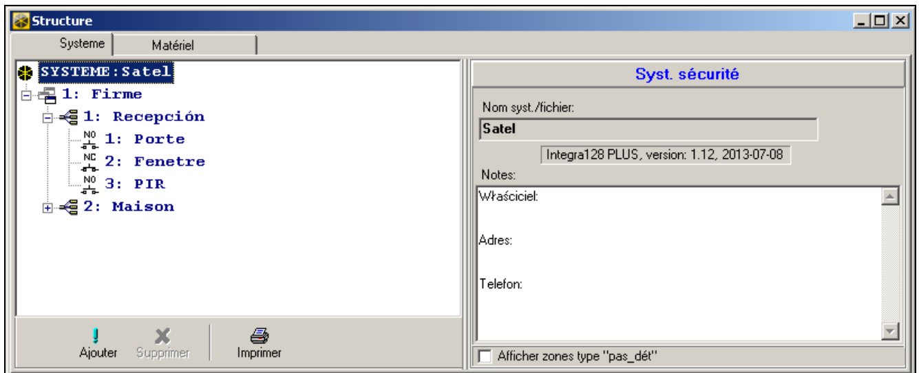
Fig. 2. Présentation de la structure du système dans le programme DLOADX.
