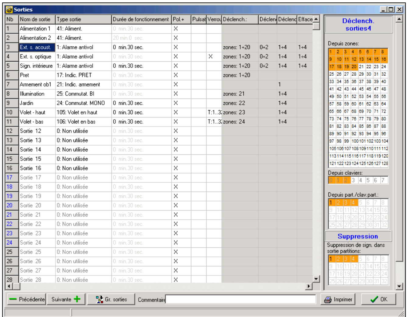
Fig. 6. Fenêtre « Sorties » dans le logiciel DLOADX.
