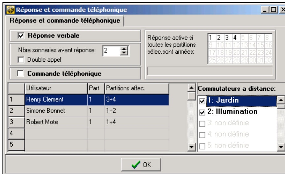
Fig. 13. Fenêtre « Réponse et commande téléphonique » dans le programme DLOADX.
