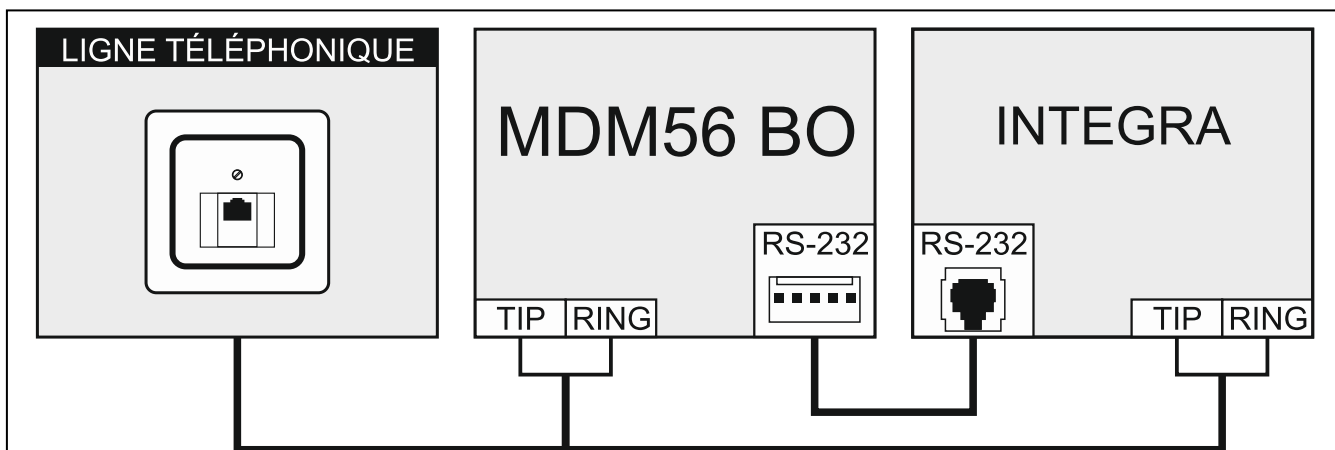
Fig. 16. Schéma de raccordement du modem MDM56 BO a la centrale.
