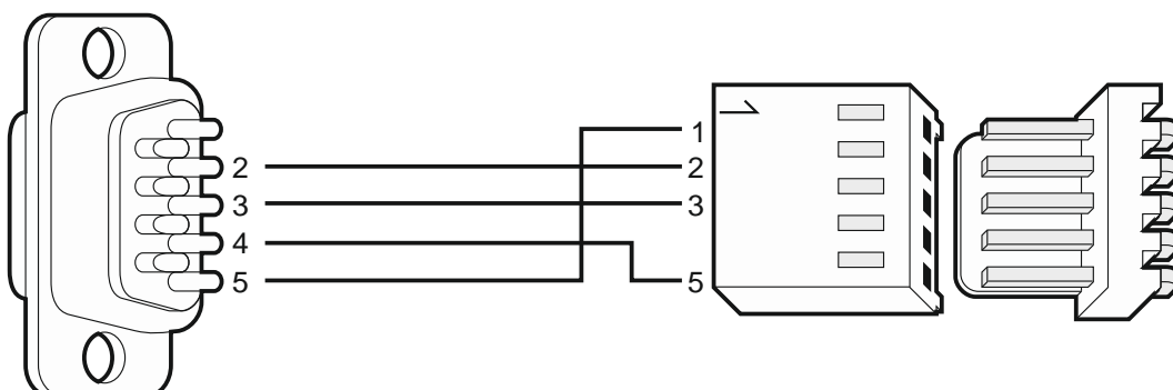
Fig. 7. Mode de raccordement de l'ordinateur au port RS-232 du clavier. À droite, la vue du connecteur dans le clavier. À gauche, le connecteur femelle DB-9 du côté des points de soudage.
