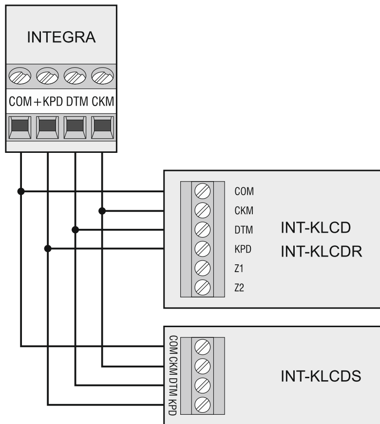
Fig. 5. Mode de raccordement des claviers (d'autres dispositifs sont raccordés de la même manière).
