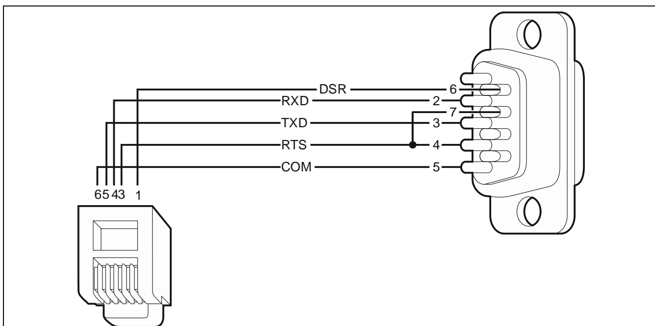
Fig. 15. Mode de raccordement des ports RS-232 de la centrale et du modem a la prise DB-9. A gauche le connecteur RJ raccordé à la prise sur la carte principale de la centrale. A droite, le connecteur male DB-9 du côté des points de soudage.
