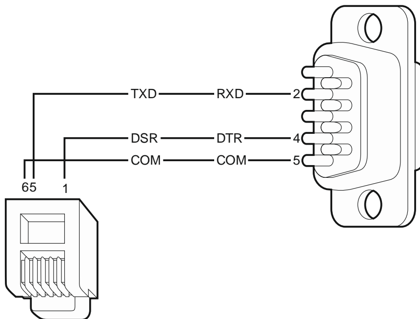
Fig. 19. Mode de raccordement de l'imprimante à l'aide de la fiche 5-pin DIN (vue de côté des points de soudure). Le connecteur RJ raccorder à la prise sur la carte principale de la centrale à gauche.
