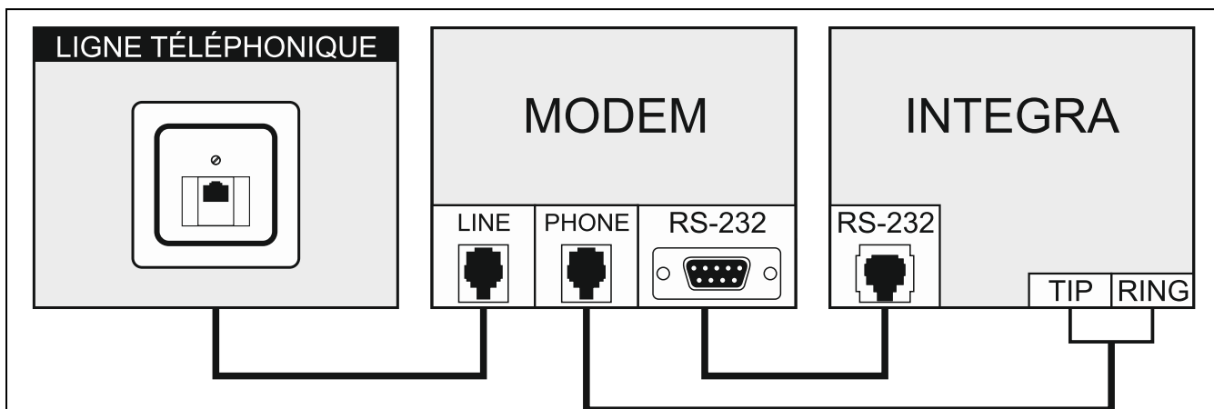
Fig. 14. Schéma de raccordement analogique du modem externe de la centrale.
