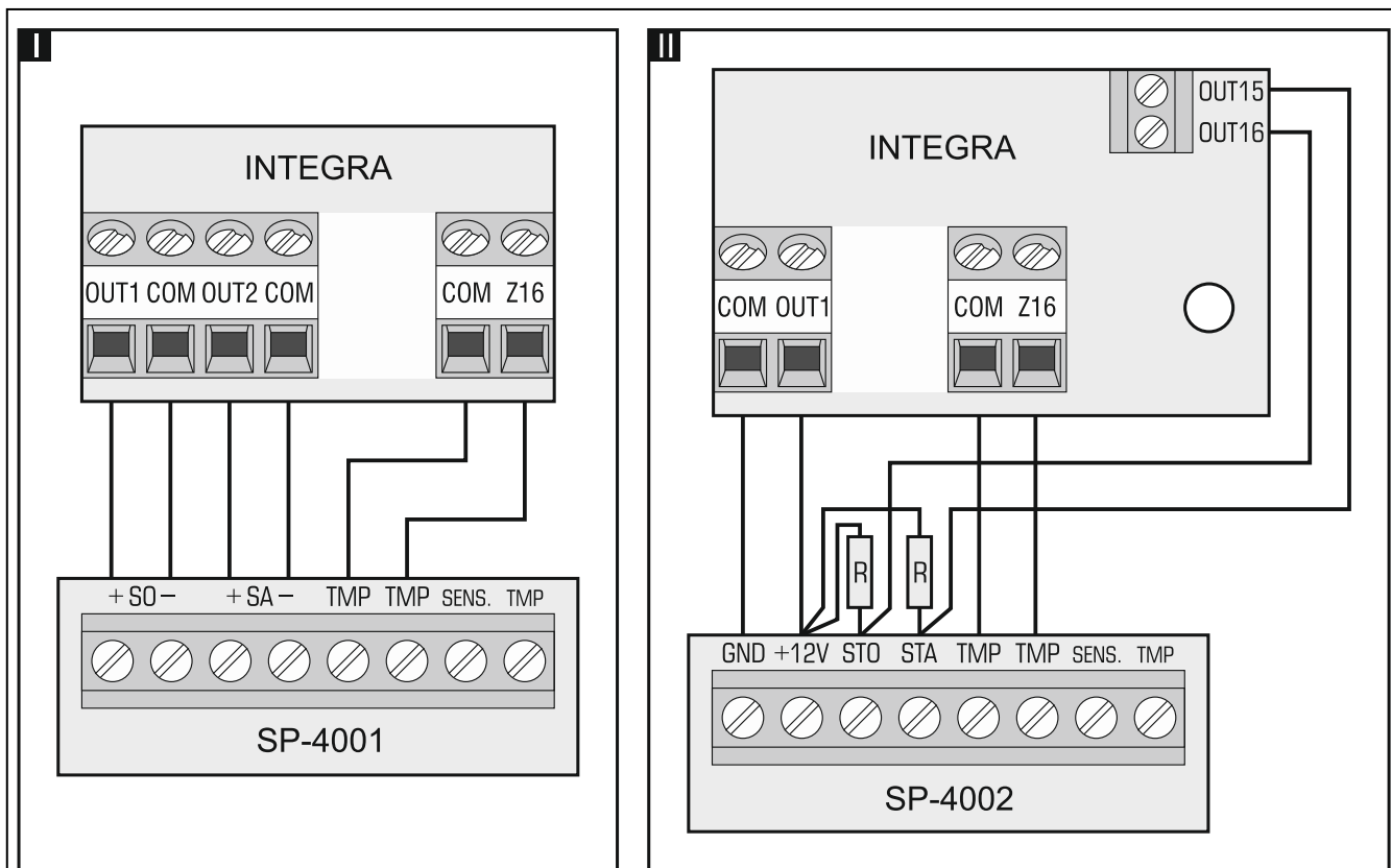
Fig. 11. Mode de raccordement des sirènes. I – sirène sans sa propre alimentation – l’alarme est signalée par les sorties à haut courant. II - sirène avec sa propre alimentation – l’alarme est signalée par les sorties à bas courant, la sortie à haut courant sert d’une sortie d’alimentation. La valeur des résistances R est de 2,2 k \Omega . Dans les deux exemples, à la zone Z16 est raccordé le circuit sabotage.
