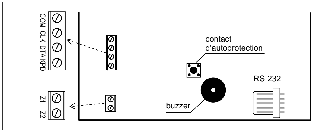
Figure 6. Vue de la carte du clavier CA-10 KLCD-L. La platine du clavier CA-10 KLCD-S diffère uniquement par dimension extérieure.
