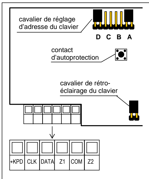
Figure 4. Vue de la carte du clavier CA-10 KLED.
