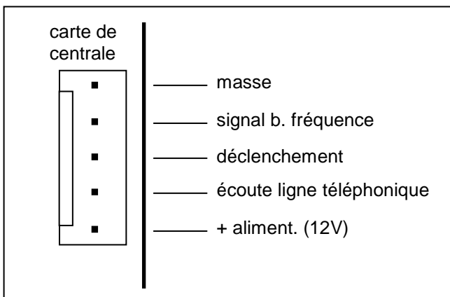
Figure 15. Connecteur raccordement de la synthèse vocale SM-2.
