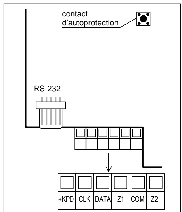
Figure 5. Vue de la carte du clavier CA-10 KLCD.
