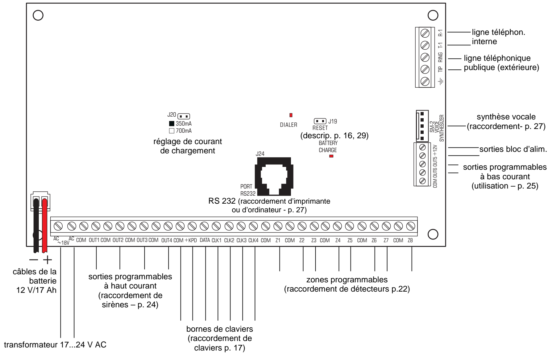
Fig. 19. Diagramme de la centrale CA-10 (description détaillées des bornes de carte principale p. 16).
