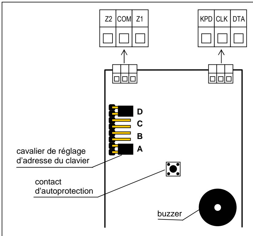
Figure 3. Vue de la carte du clavier CA-10 KLED-S
