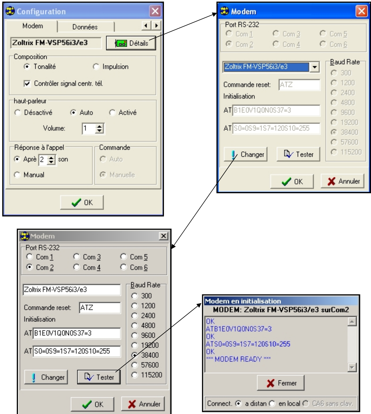
Figure 18. Fenêtres de dialogue du logiciel DLOAD10.
