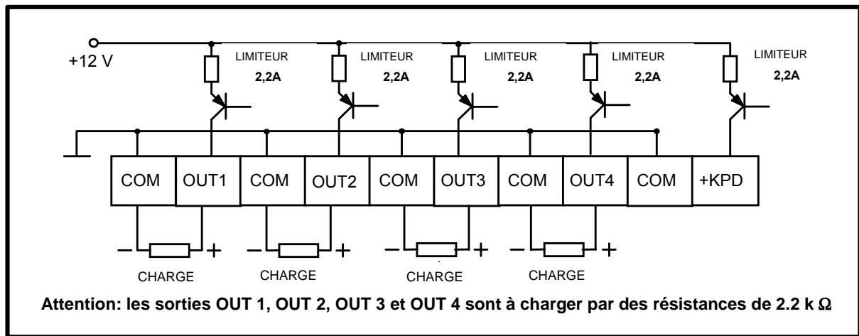
Figure 12. Schéma de sorties à haut courant.
