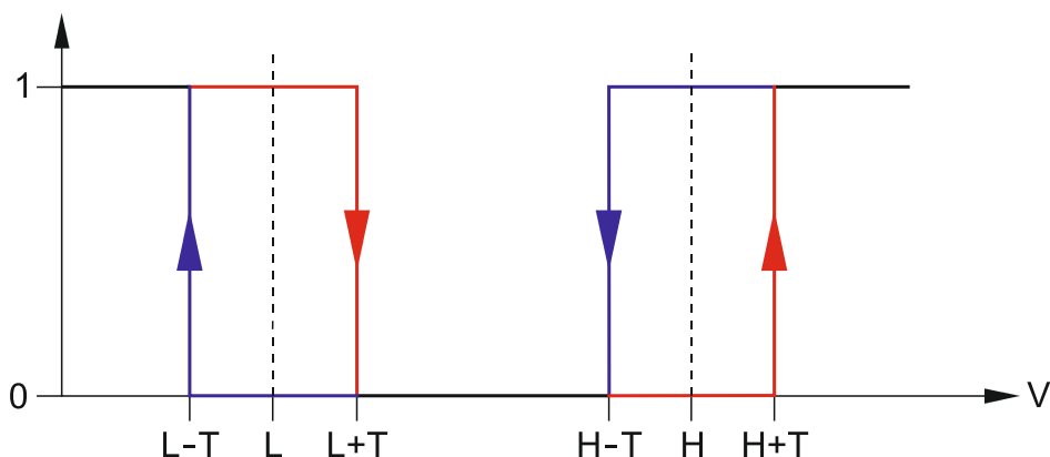
Obr. 11. Chování analogového vstupu v provozu. 0 – bez narušení. 1 – narušení. L-T – záporná tolerance prahu L. L – práh nízkého napětí. L+T – kladná tolerance napětového prahu L. H-T – záporná tolerance napětového prahu H. H – vyšší úroveň napětí. H+T – kladná tolerance napětového prahu H.
