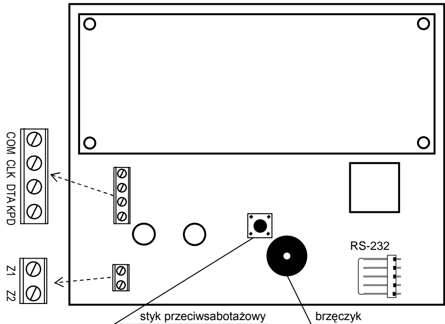
Rysunek 2. Schematyczny widok płytki manipulatora wraz z oznaczeniem zacisków przewodów (wersja wykonania LCD-L V1.1).
