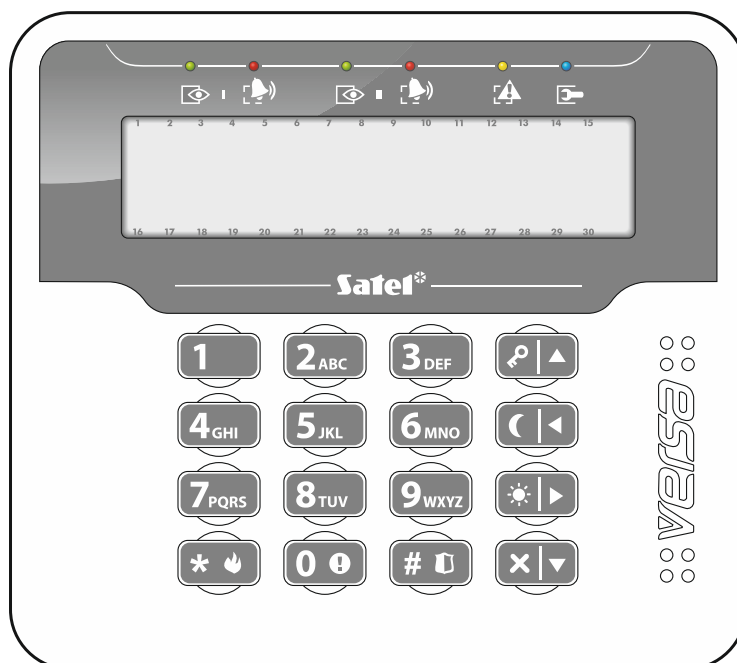
Abb. 1. Bedienteil VERSA-LCDM (Bedienteile VERSA-LCDR, VERSA-KWRL2 und VERSA-LCDM-WRL unterscheiden sich nur durch einige graphische Elemente auf dem Frontteil).
