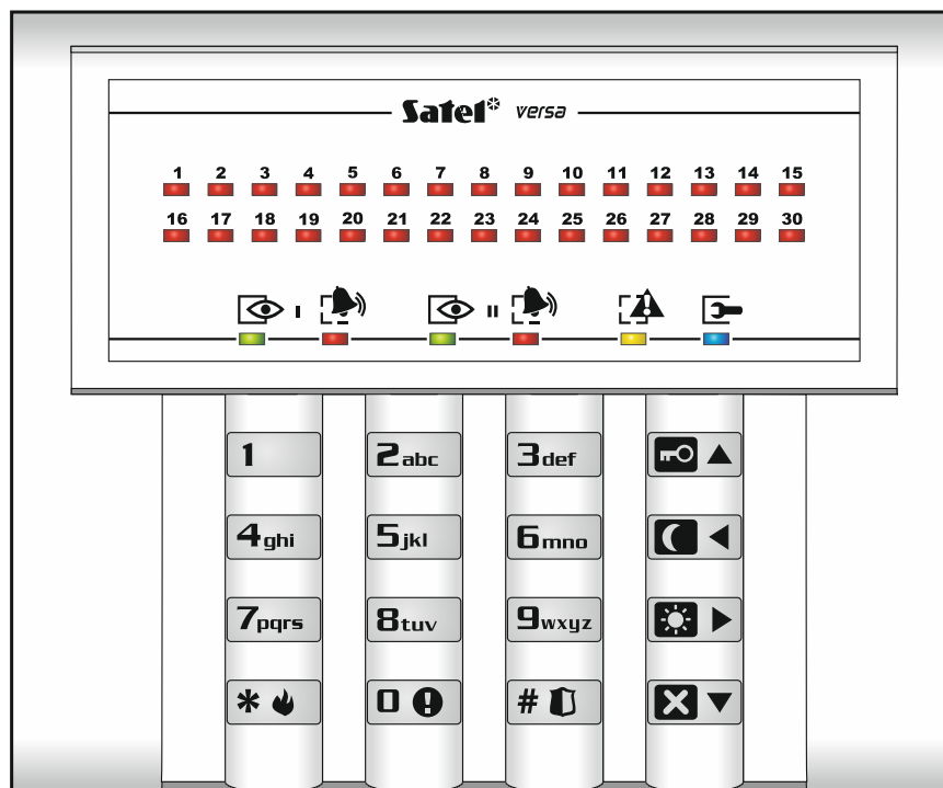
Abb. 1. Bedienteil VERSA-LED.
