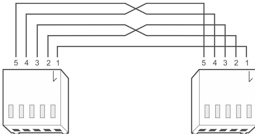
Abb. 6. Kabel zur Verbindung der RS-232-Schnittstelle des Moduls INT-GSM LTE und einer INTEGRA-Zentrale mit der PIN5-Buchse.
