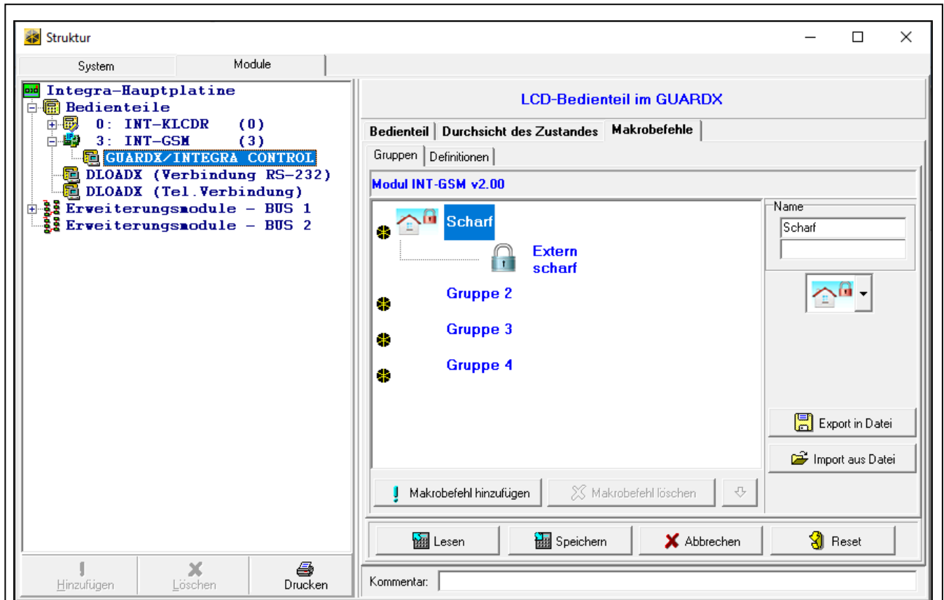
Abb. 18. Programm DLOADX: Registerkarte „Gruppen“.
