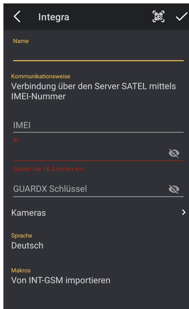
Abb. 24. INTEGRA CONTROL App (Android System): Bildschirm zum Hinzufügen der Alarmzentrale.
