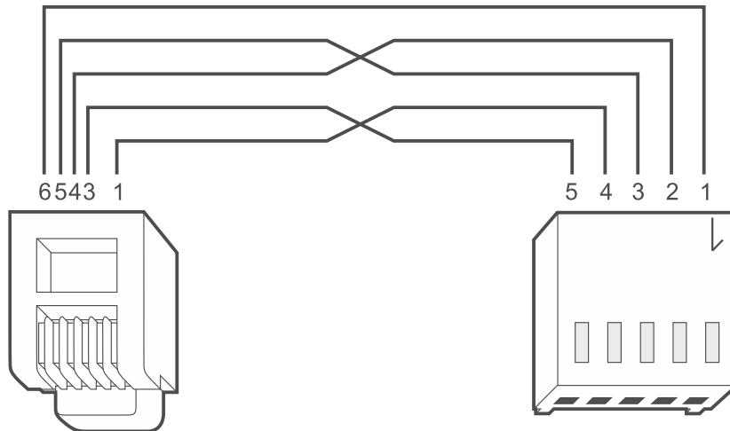
Abb. 5. Kabel zur Verbindung der RS-232-Schnittstelle des Moduls INT-GSM LTE und einer INTEGRA / INTEGRA Plus Zentrale mit der RJ-Buchse.
