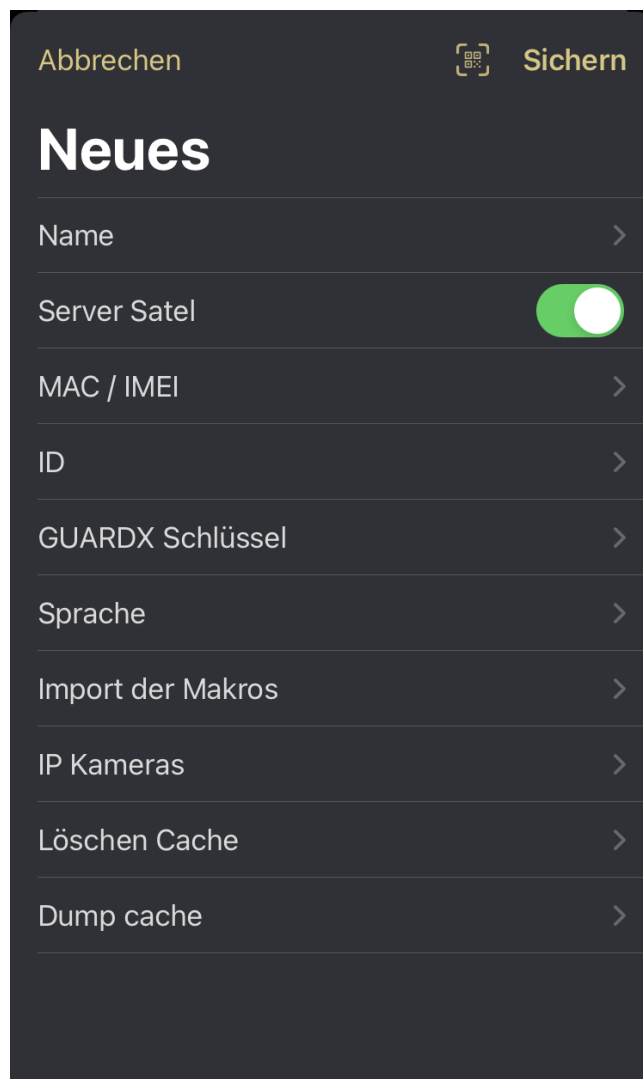
Abb. 26. INTEGRA CONTROL App (System iOS): Bildschirm zum Hinzufügen der Alarmzentrale.
