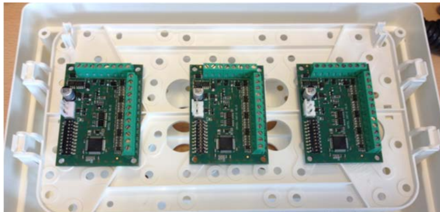
OPU-3 met 3x INT-E
