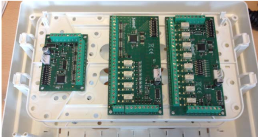
OPU-3 met INT-O, INT-PP en INT-E
