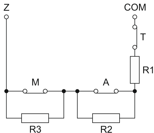
Fig. 4. Nummering van EOL weerstanden. T – sabotage. A – alarm. M – maskering. Voor de EOL en 2EOL configuraties is de R3 weerstand irrelevant. Voor de EOL configuratie is de weerstandswaarde de som van de waarden als geprogrammeerd bij de R1 en R2 weerstanden.
