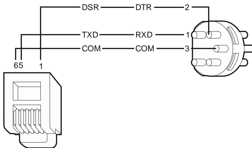
Fig. 18. Printer aansluiting met gebruik van een DIN 5-pin plug (aanzicht soldeer zijde). Links weergegeven is de RJ connector welke aangesloten wordt op de RJ aansluiting van de hoofdprint.
