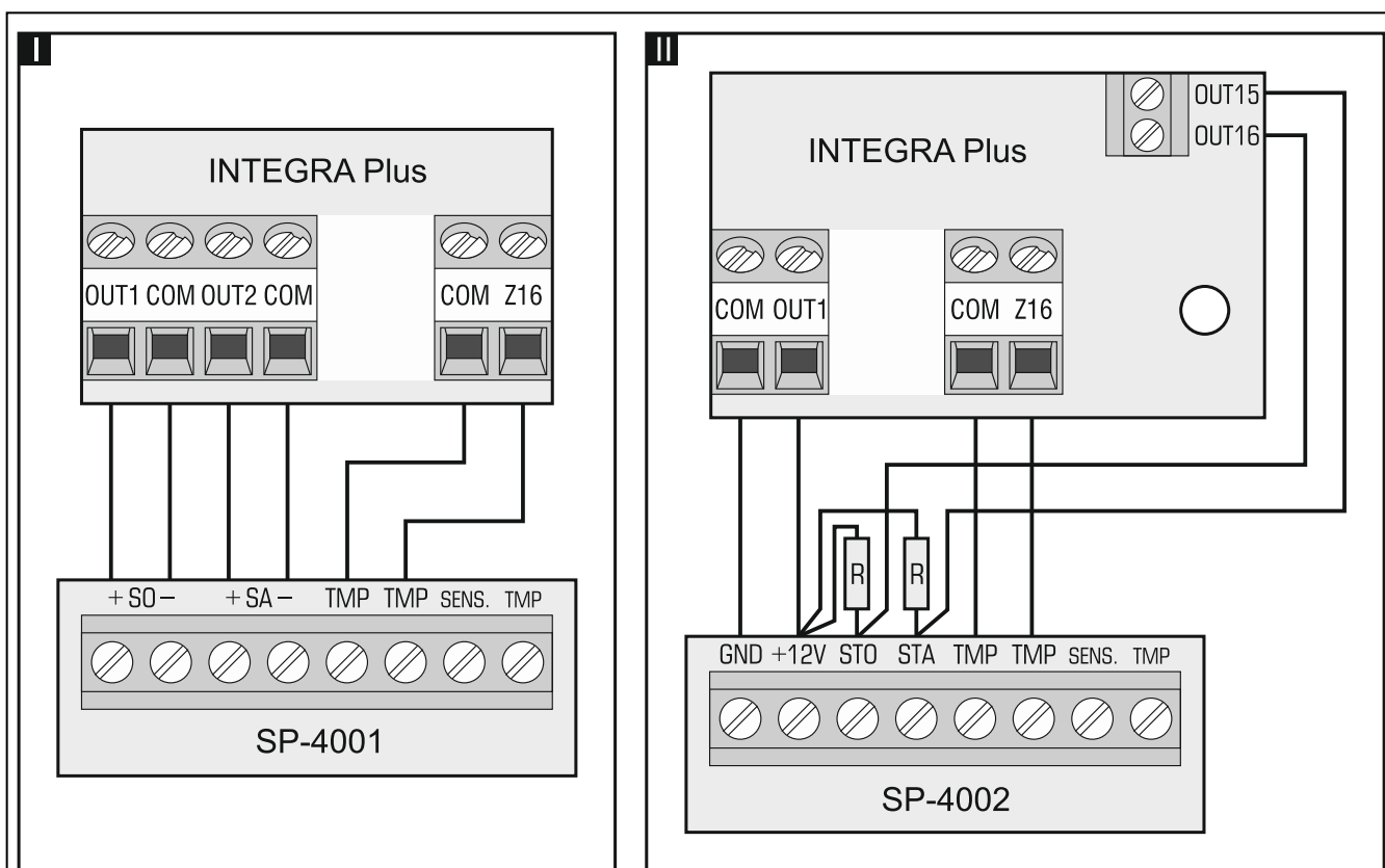
Fig. 9. Sirene aansluitvoorbeeld. I – sirene zonder eigen voeding – alarm signalering wordt aangestuurd door de hoogvermogen uitgangen. II - sirene met eigen voeding – alarm signalering wordt aangestuurd door de laagvermogen uitgangen waarbij de hoogvermogen uitgang dient als voedingsuitgang. De weerstandswaarde van R is 2.2 kΩ. In beide gevallen is de sabotage aangesloten op zone Z16.
