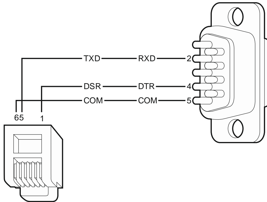
Fig. 17. Printer aansluiting met gebruik van de DB-9 male plug (aanzicht soldeer zijde). Links weergegeven is de RJ connector welke aangesloten wordt op de RJ aansluiting van de hoofdprint.
