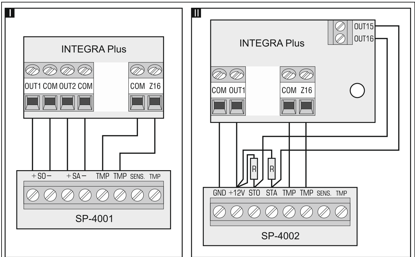
Fig. 9. Mode de raccordement des sirènes. I – sirène sans sa propre alimentation – l’alarme est signalée par les sorties à haut courant. II - sirène avec sa propre alimentation – l’alarme est signalée par les sorties à bas courant, la sortie à haut courant sert d’une sortie d’alimentation. La valeur des résistances R est de 2,2 k \Omega . Dans les deux exemples, à la zone Z16 est raccordé le circuit sabotage.
