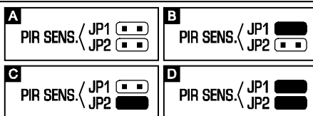
Fig. 2. Método para el ajuste de sensibilidad del detector (A – baja sensibilidad, B y C – media sensibilidad, D – alta sensibilidad) [●●●● – pins cerrados; □□□□ – pins abiertos].
