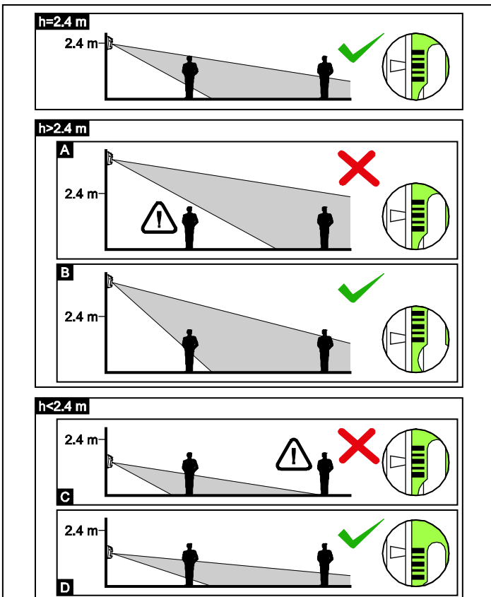
Fig. 7. Influencia de la altura de montaje en el área observada por el detector y el método de posicionamiento de la placa base para optimizar esta área. Dependiendo de la altura de instalación la mediana línea de la escala debe encontrarse: en frente del indicador en la caja (altura de montaje 2,4 m), por encima del indicador (altura de montaje superior a 2,4 m – ejemplo B) o debajo del indicador (altura de montaje no superior a 2,4 m – ejemplo D).
