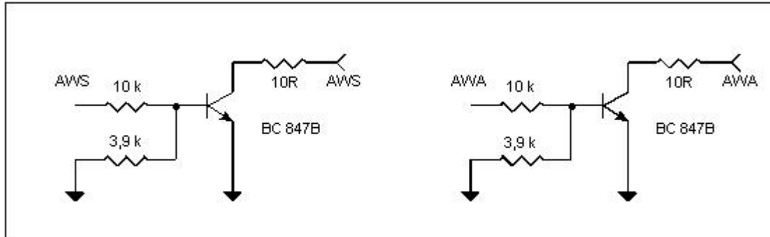
Fig. 2. Esquema de salidas AWS y AWA.
