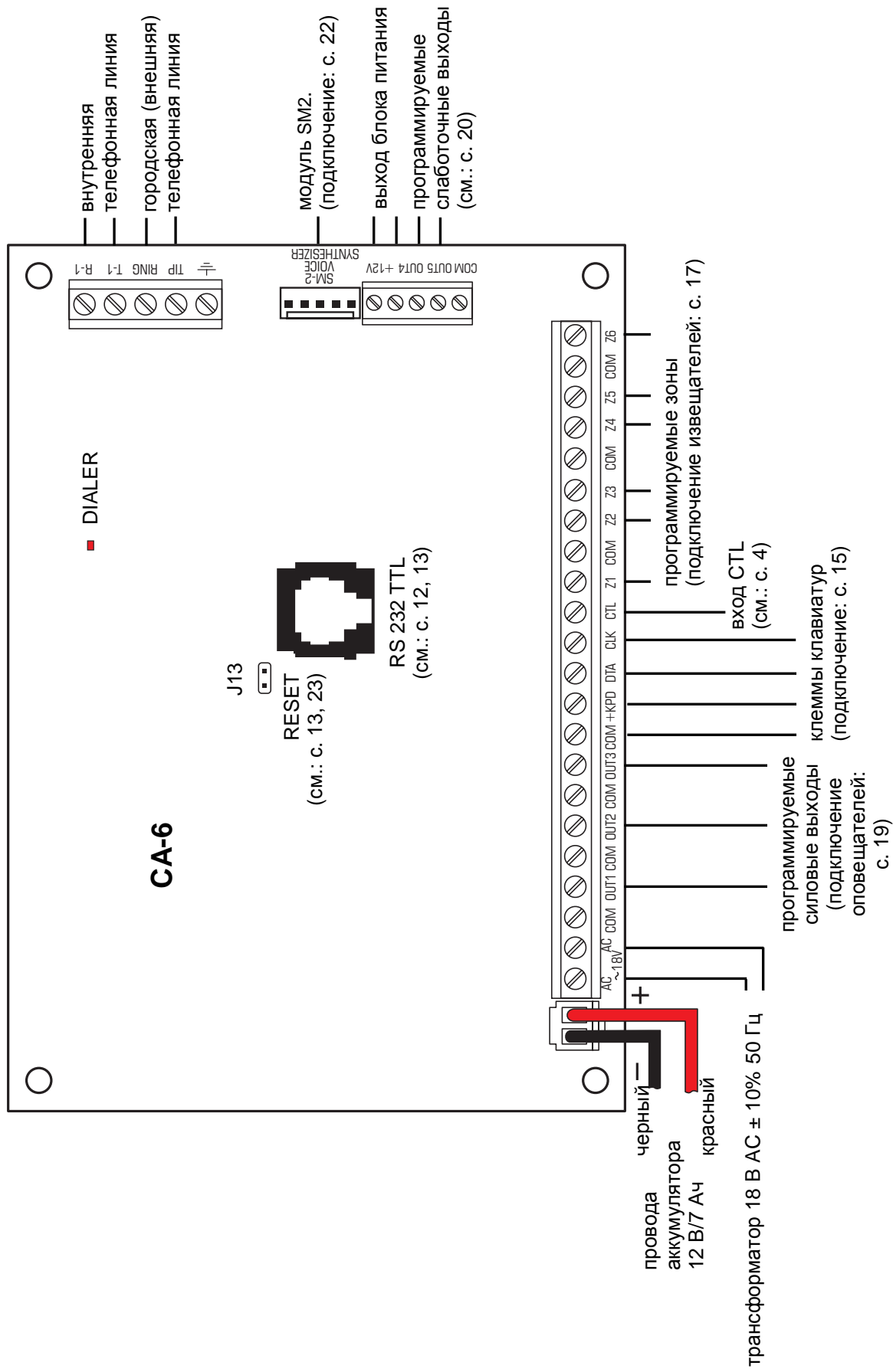
Схематичный вид приемно-контрольного прибора SA-6 (детальное описание клемм основной платы см.: с. 14).
