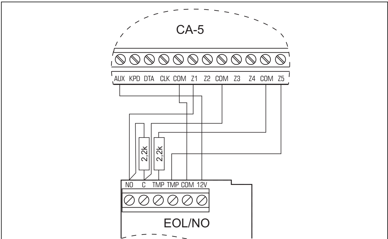
Рис. 8. Пример подключения к ПКП извещателя по схеме с оконечным резистором EOL/NO.
