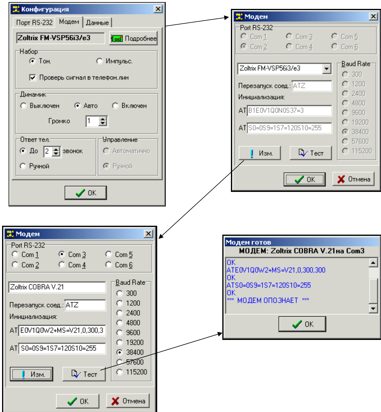
Рис. 13. Окна диалогов программы DLOAD10.
