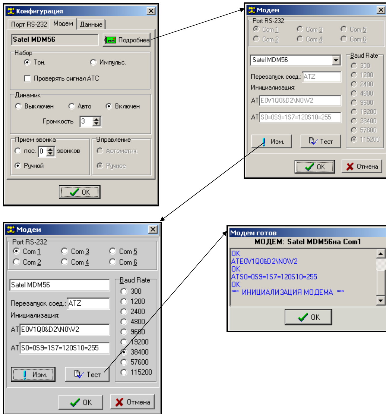
Рис. 18. Окна диалогов программы DLOAD10
