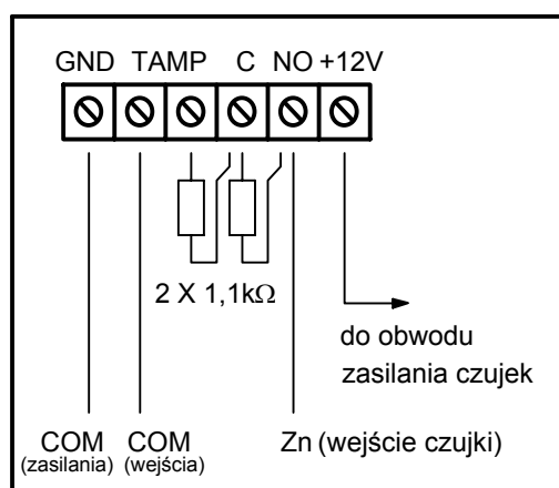
Rys. 4 - Podłączenie czujki 2EOL
