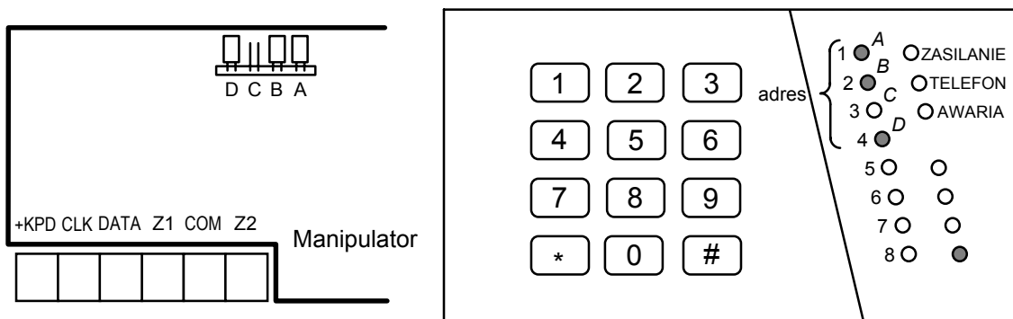
Rys.11 - Ustawienie zworek i odpowiadające im diody przy programowaniu.
