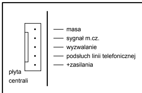
Rys.8 - Opis gniazda do podłączenia syntezeru mowy SM-2.
