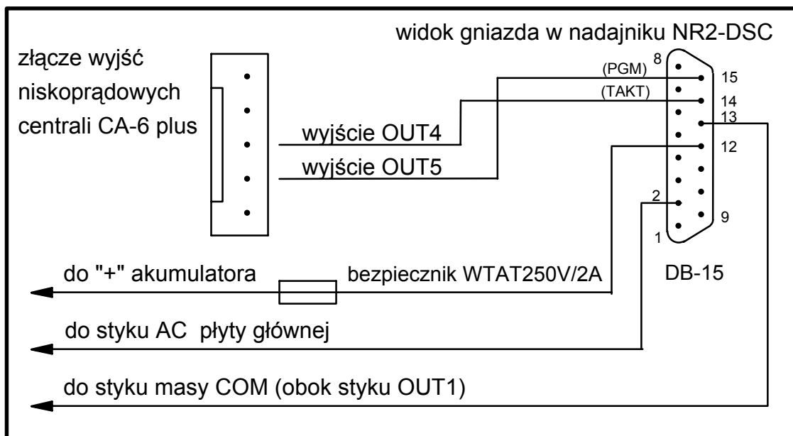
Rys.7 - Podłączenie nadajnika sterowanego typu NR2-DSC firmy NOKTON s.c.
