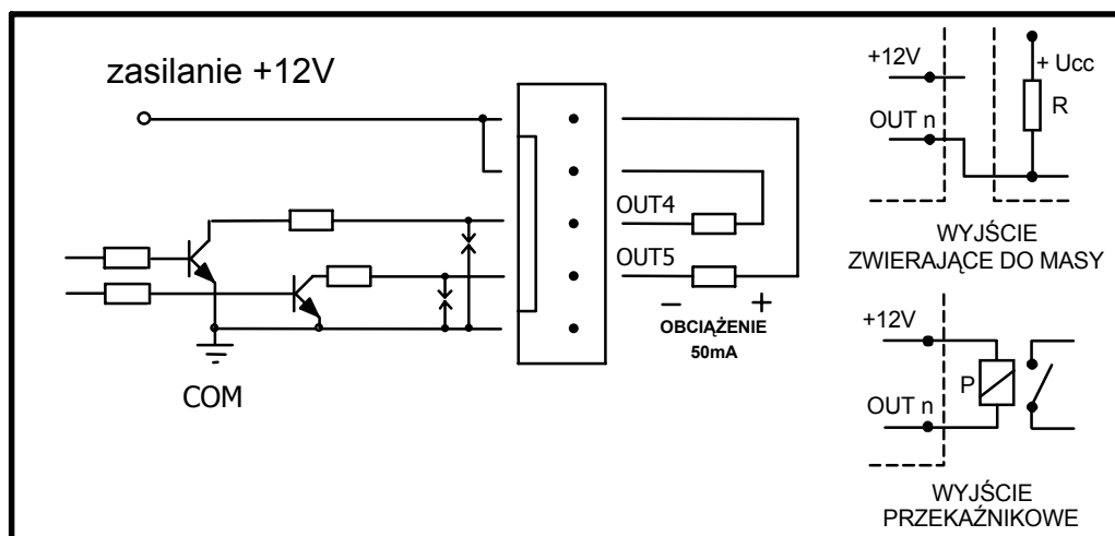
Rys.6 - Schemat wyjść niskoprądowych OUT4 i OUT5 i podłączenie obciążenia.
