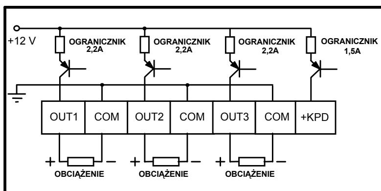
Rys.5 - Schemat wyjść wysokoprądowych.
