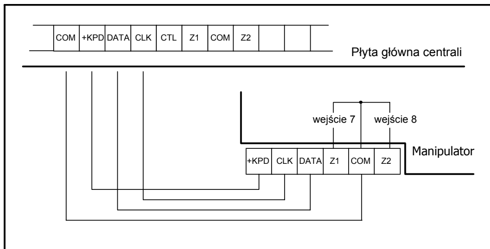
Rysunek 3. - Sposób podłączenia manipulatora do centrali.
