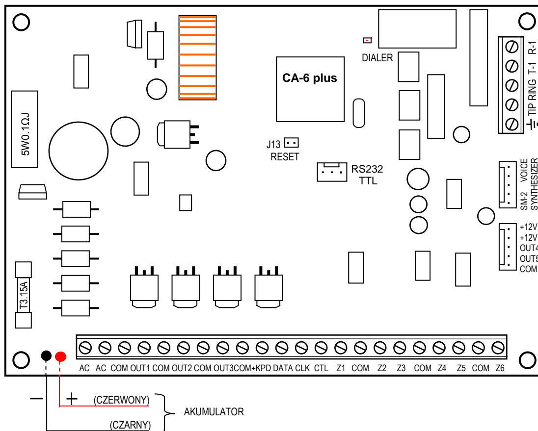
Rysunek 1. - Widok schematyczny płyty centrali CA-6 plus wykonanej w wersji CA6P V4.1.
