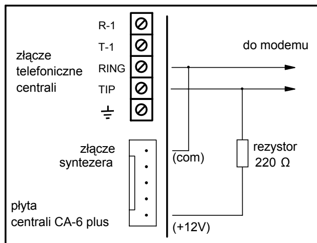
Rys.12 - Podłączenie centrali do modemu przy programowaniu lokalnym.
