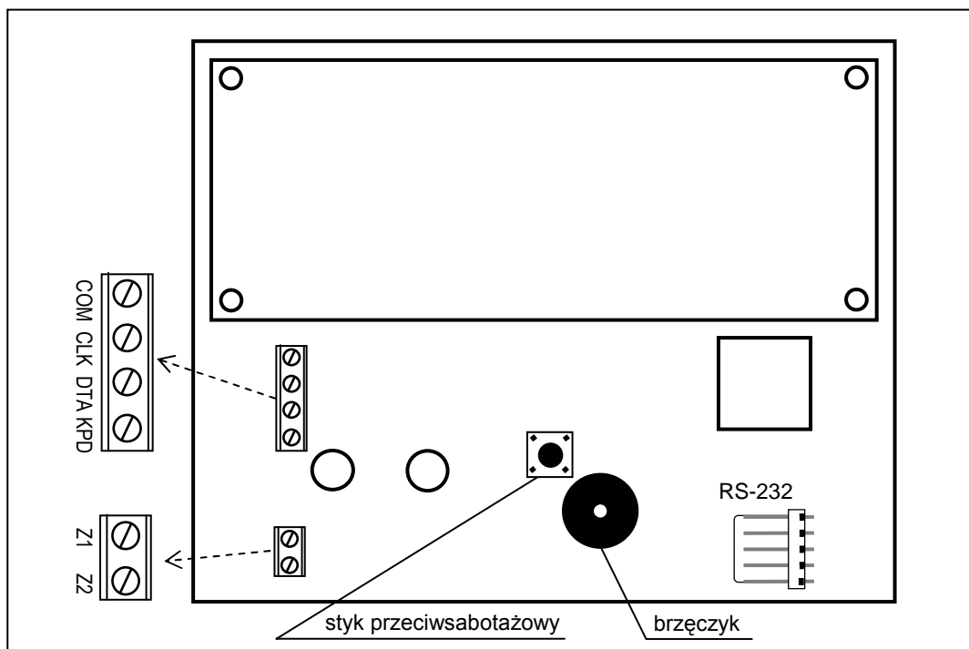
Rysunek 5. Widok płytki manipulatora CA-10 KLCD-L wraz z oznaczeniem zacisków przewodów. Płytki manipulatora CA-10 KLCD-S różni się jedynie rozmiarem zewnętrznym.
