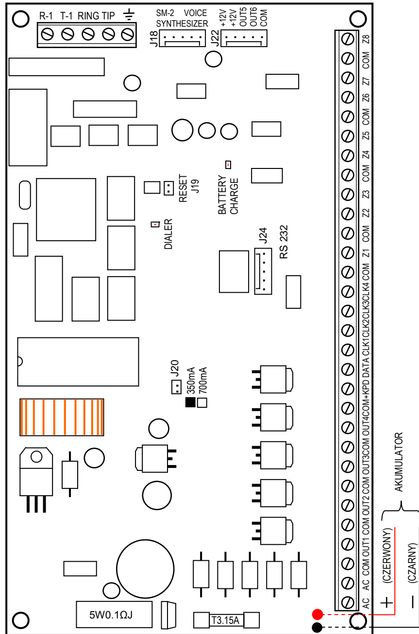
Rysunek 1 Widok schematyczny płyty centrali w wykonaniu CA10PV4.3.
