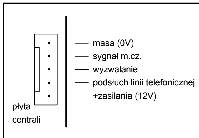
Rys. 13. Gniazdo do podłączenia syntezera mowy SM-2.
