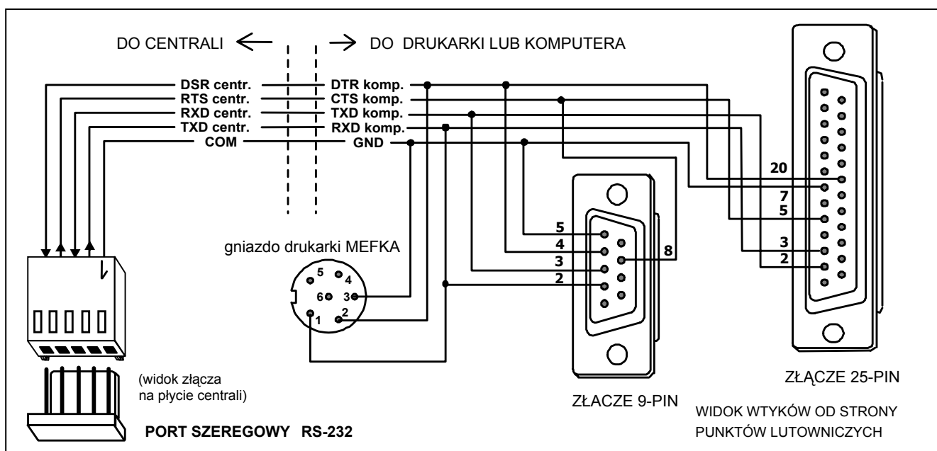
Rys. 14. Sposób podłączenia drukarki lub komputera do portu RS-232 centrali.
