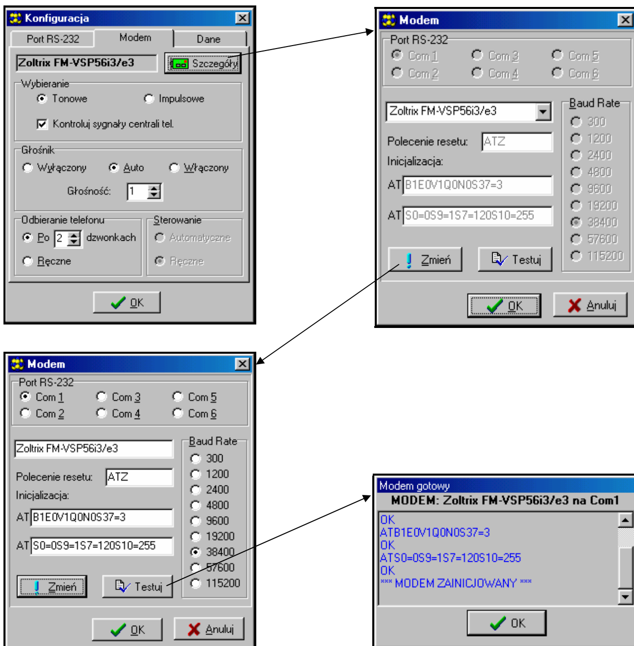
Rysunek 15. Okna dialogowe programu DLOAD10.
