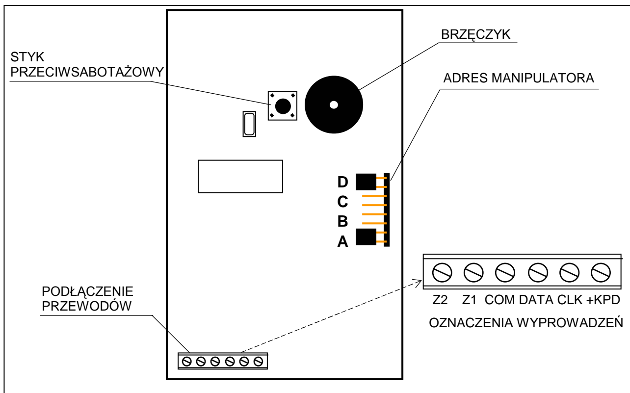
Rysunek 6. Widok płytki manipulatora CA-10 KLED-M.
