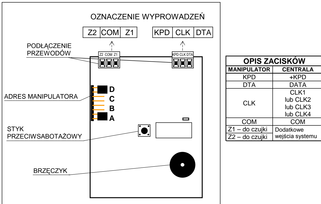
Rysunek 7. Widok płytki manipulatora CA-10 KLED-S.
