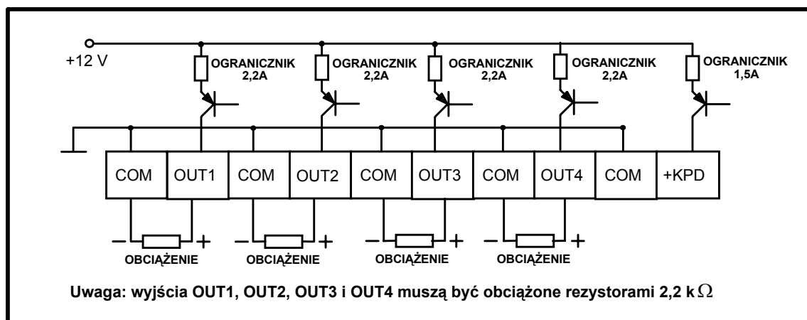
Rysunek 10. Schemat wyjść wysokoprądowych.
