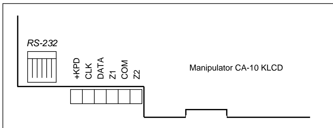
Rysunek 4. Widok złącz manipulatora CA-10 KLCD
