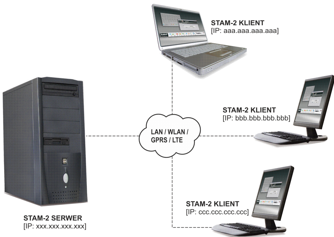
Rys.4. Przykładowa konfiguracja stacji monitorującej STAM-2.
